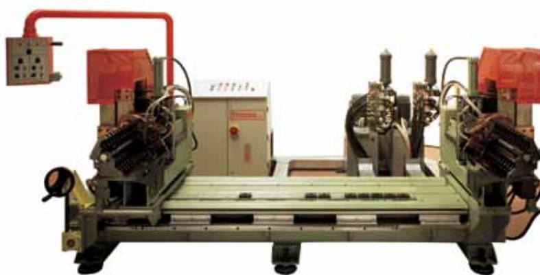
Complesso di assemblaggio e riscalcatura componenti di riscaldamento Assembly for heating component mounting and upsetting
