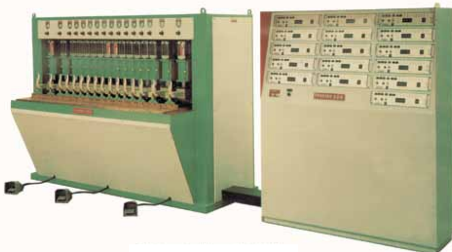
Saldatrice con unità multipli indipendenti Welding machine with independent multiple units
